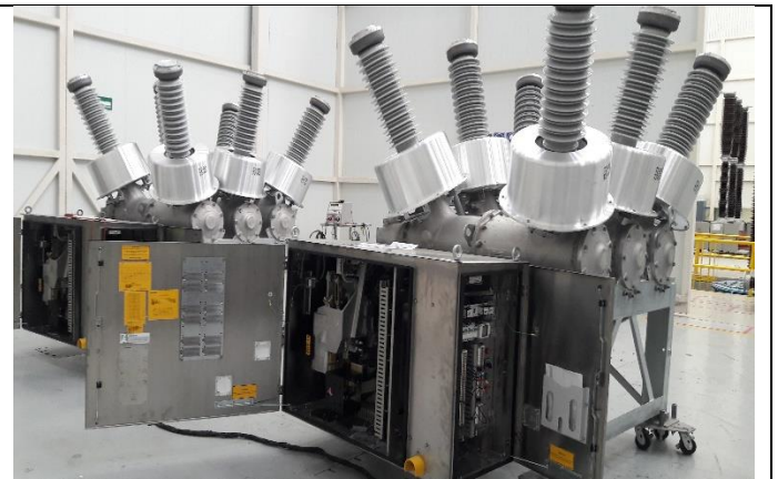
Foto # 2, Inspección del gabinete de los interruptores de 34,5 kV en fábrica.
