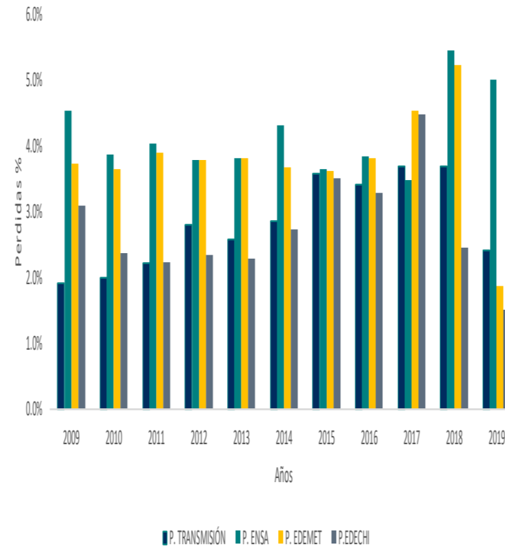
PERDIDAS DE ENERGÍA TOTALES
