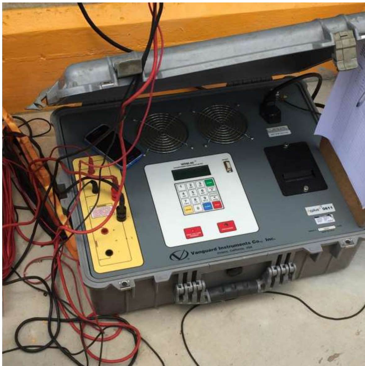
Equipo de Pruebas para medir resistencia de devanado al transformador
