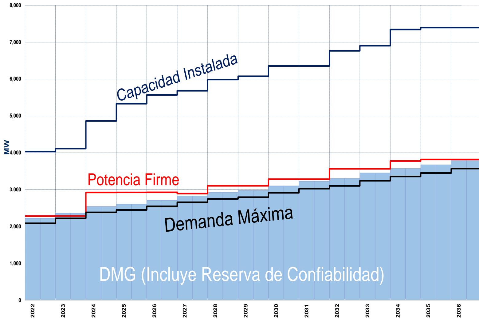
Gráfico N° A1.1 Balance de Potencia vs Demanda del Escenario Tendencial
