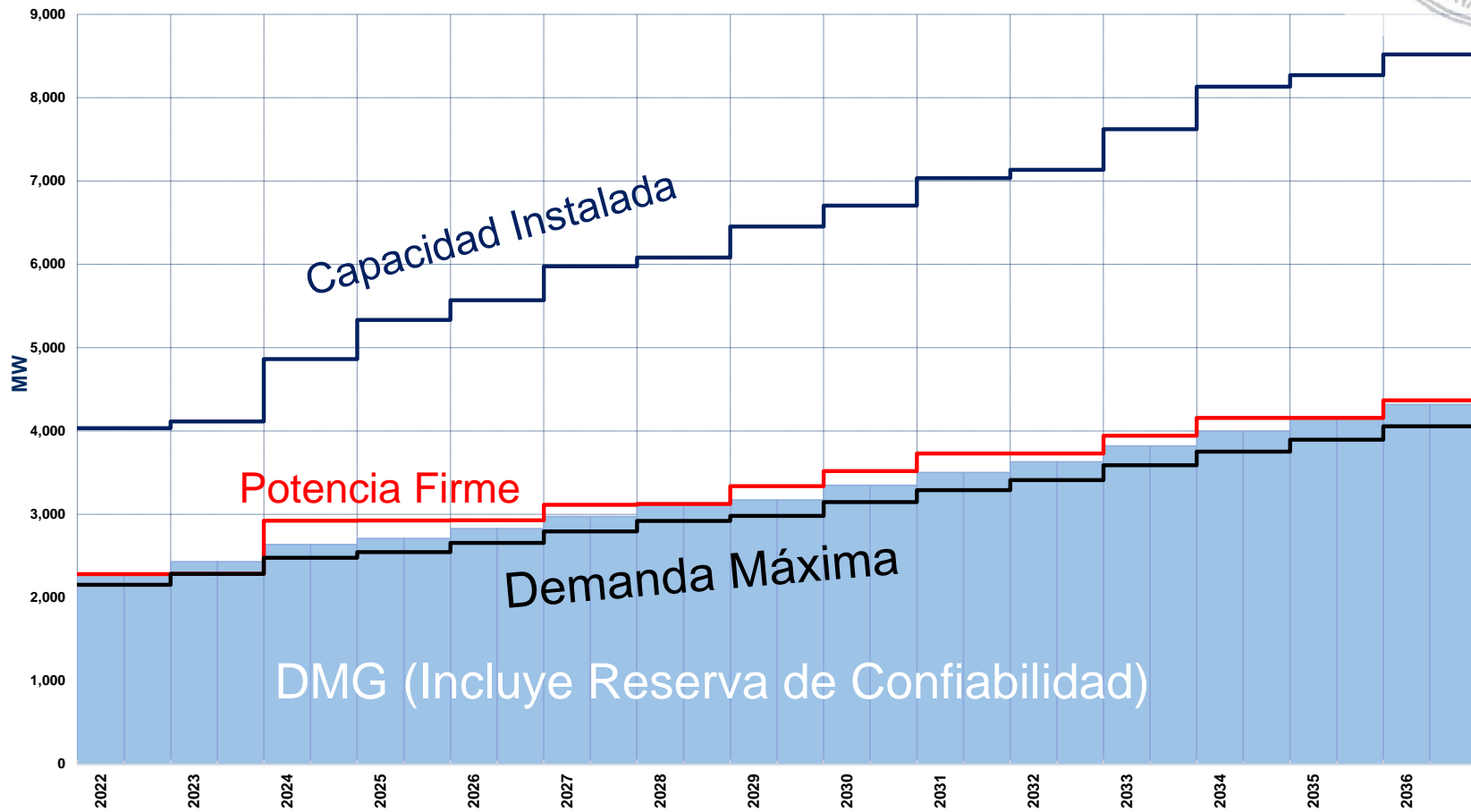
Gráfico N° A2.1 Balance de Potencia vs Demanda del Escenario Alternativo I
